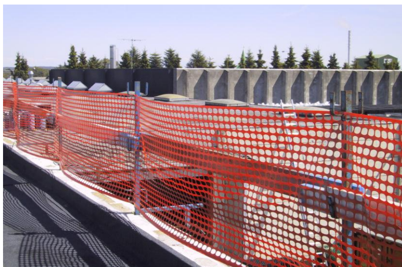
Afspærringsnet type F23 monteret på byggeplads sammen med sikkerhedsstakit giver en tydelig afspærring.
